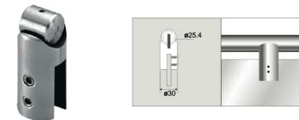
DR8200E-14 ■ Conector de Tubo de Ø25.4mm en ángulo
