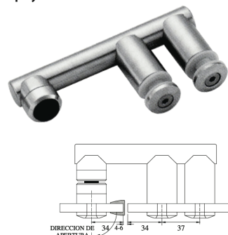
DR8200E-8 ■ Tope y conector de 180°
