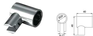
DR8200E-11 ■ Conector de Fijación de Tubo de Ø20mm a muro
