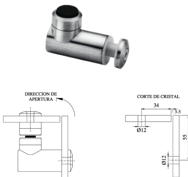
DR8200E-8 ■ Tope y conector de 180°
