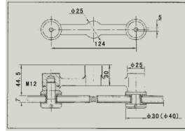
Conector de Series Fs para Barandas
