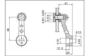
Conector de Series Fs para Barandas
