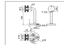
Conector de Series Fs para Barandas
