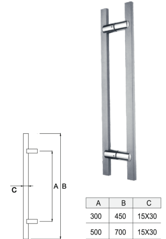
DH-117 ■ Tirador Material: Aleación de Zinc Acabado: Satinado
