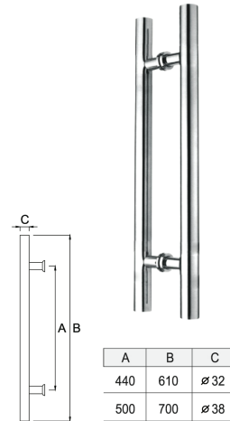
DH-115 ■ Tirador
