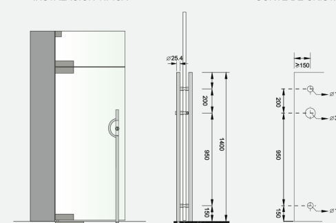
INSTALACION TIPICA
