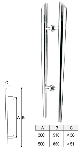
DH-110 ■ Tirador
