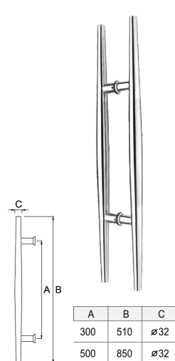
DH-112 ■ Tirador
