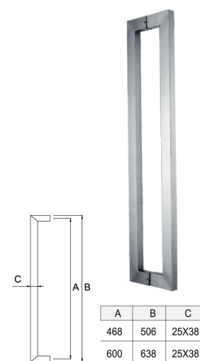
DH-115 ■ Tirador
