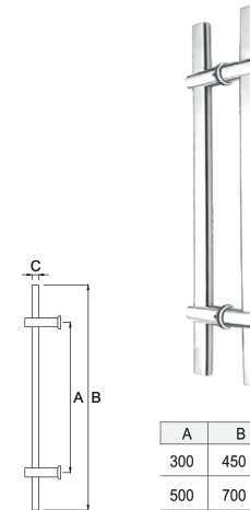
DH-116 ■ Tirador
