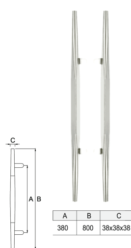
DH-111 ■ Tirador
