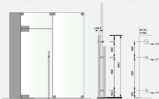
INSTALACION TIPICA
