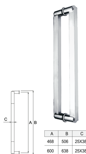
DH-116 ■ Tirador
